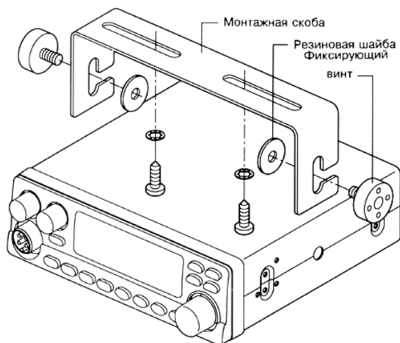
Рис. 2. Крепление радиостанции при помощи монтажной скобы.
