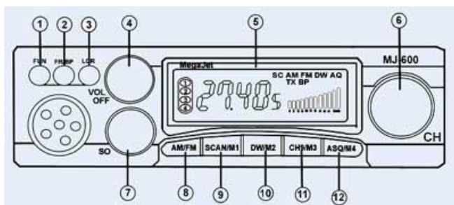
Рис. 1. Органы управления и отображения MJ-600
