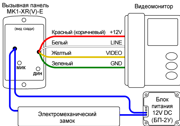
Рис 1. Подключение блока вызова MK1-XRV-E
