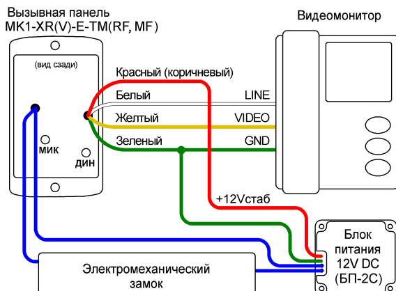
Рис 2. Подключение блока вызова MK1-XRV-E-TM(RF, MF)
