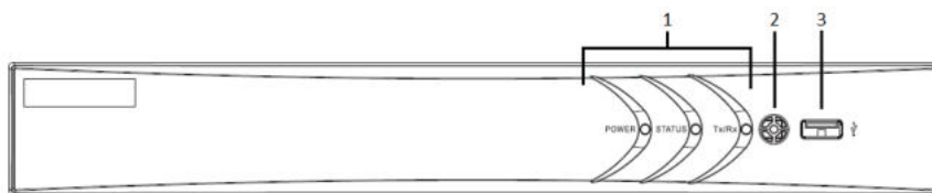
Рисунок 1-2 Передняя панель 2
