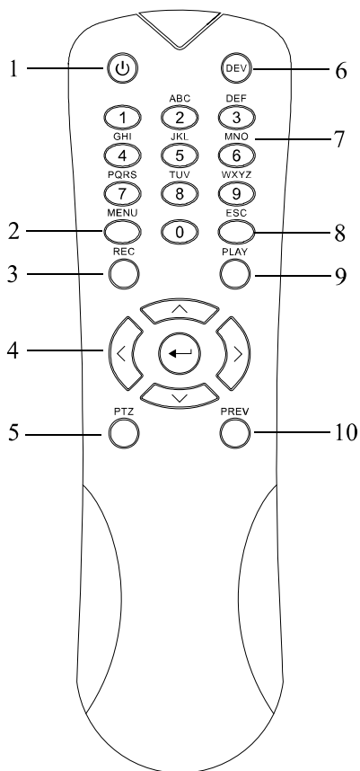
Рисунок 1-3 Пульт управления
