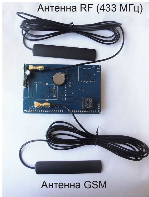
Внешняя антенна
