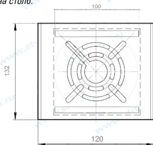
Рис.1 Габаритные размеры
