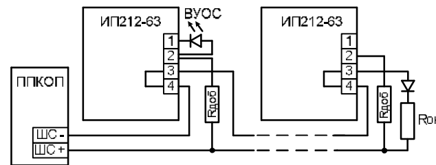
Рис.2 Типовая схема включения извещателя для приборов с переполюсовкой шлейфа сигнализации. Величина резисторов R_{ок} и R_{доб} определяется в соответствии с техническим описанием ППКОП
