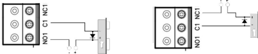
Рис. 16. Подключение замков при использовании внешнего источника питания
