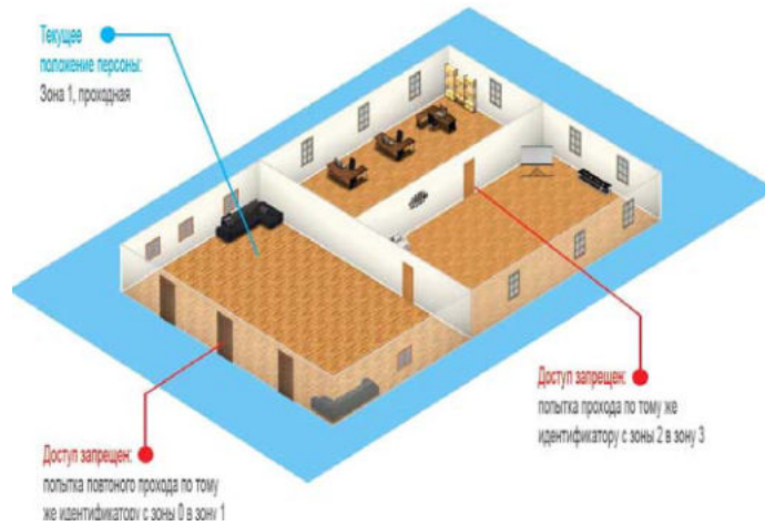
Рис 7. Отслеживание нарушений
