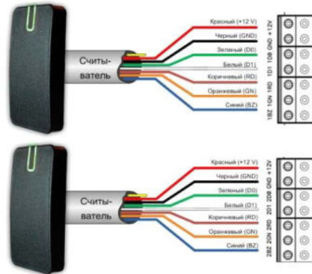
Рис.11. Подключение считывателей
