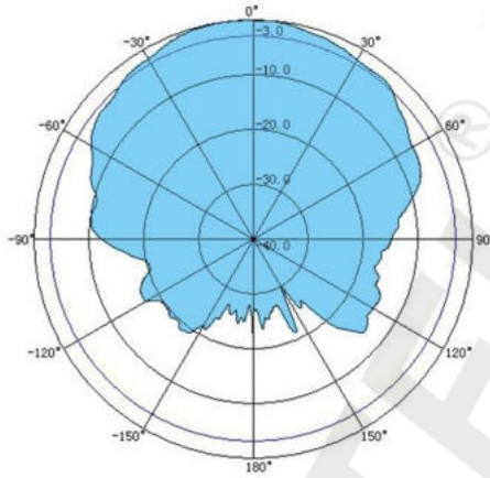
ГОРИЗОНТАЛЬНАЯ ПЛОСКОСТЬ
