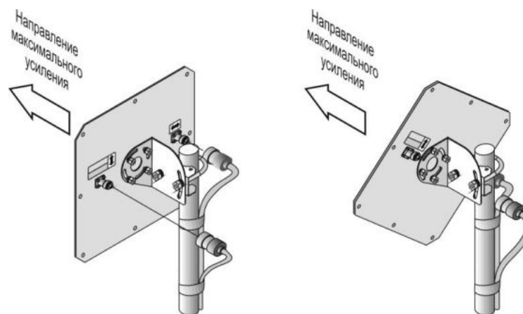
Рисунок 2. Сборка антенны
