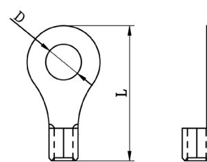
Круглая клемма:
