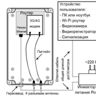
Пример размещения оборудования в гермобоксе
