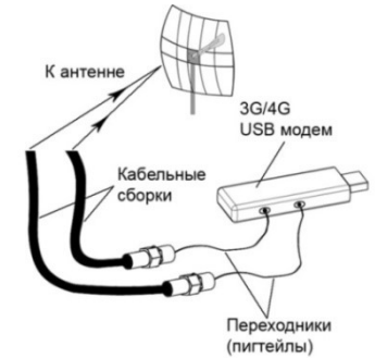
Пример подключения 3G/4G USB модема
