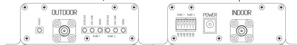
Рисунок 2 – Панели усилителя
